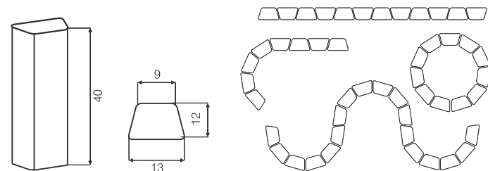
Wymiarowanie.
