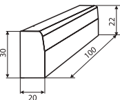
Krawężnik skośny lewy/prawy
