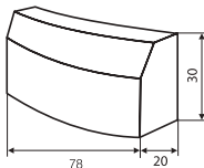
Krawężnik łukowy R - 6 m 48 szt. na okrag
