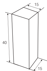
Palisada 40 ok. 7 szt na m b.
