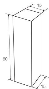
Palisada 60 ok. 7 szt na m b.
