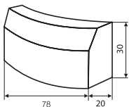
Krawężnik łukowy R - 1m 8 szt. na okrag
