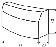
Krawężnik łukowy R - 3 m 24 szt. na okrag
