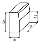
Krawężnik półowka
