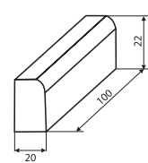
Krawężnik najazdowy
