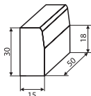
Krawężnik połówka
