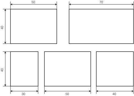
Schemat ułożenia elementów na palecie.
